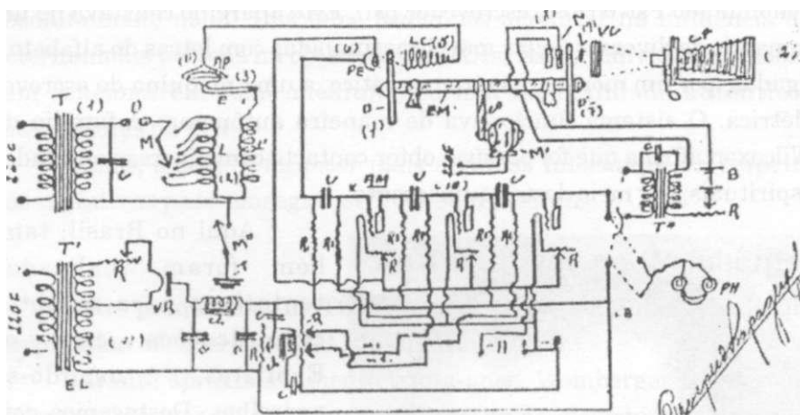
Esquema do projeto do aparelho criado pelo brasileiro Próspero Lapagesse, destinado à TCI com o Além. (Extraído da Revista Internacional de Espiritismo , maio de 1933)
