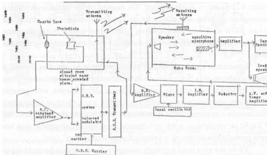
Projeto de aparelho eletrônico para TCI com o Plano Espiritual, de autoria do prof. J. B. Shikalgar, do Poona College, em Poona -1, Índia. (Extraído da revista Indiana Life-Beyond , vol. III, n. 10, julho 1983)
